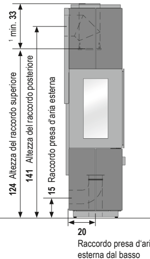
Vista laterale Maiolica/Pietra naturale:
