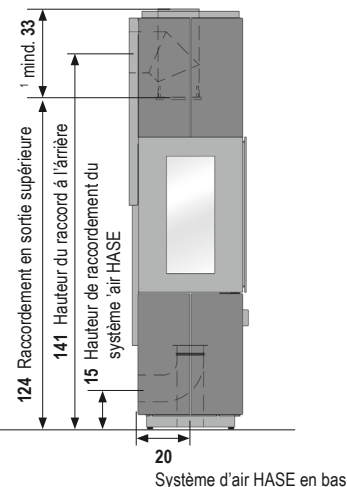
Vue de côté Céramique/Pierre naturelle:
